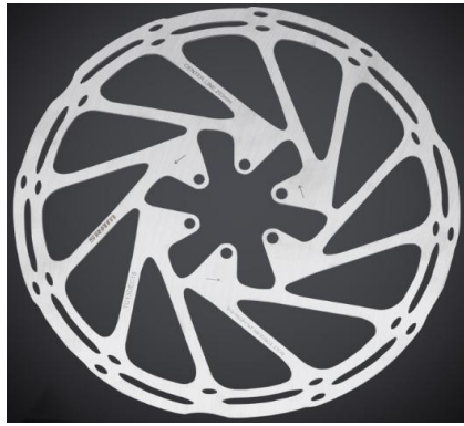
Centerline disc rotor 203mm
